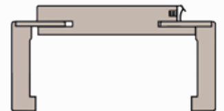
Sinus 75 E
