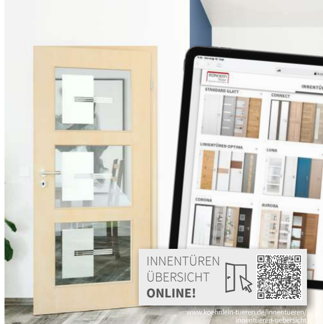
STANDARD GLATT CPL Ahorn-Reproduktion, Design-LA 3R, Zarge KÖNOSOFT, Drückergarnitur Merida, Edelstahl, Rosette rund, Verglasung: Oros WT, Grundfläche klar, Linien sandgestrahlt, Ausführung Dreifach-Linie, Ausführung Cambio Centro schlosseitig, Rand 50 klar
