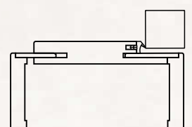
Zarge Sinus stumpf einschlagend
